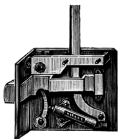
No. 93 med Spiralfjedre.
