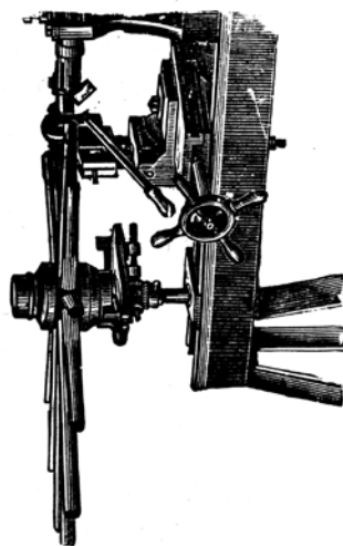
(Tilhørende ovenstaaende Maskine til Hjulfabrikation.)
