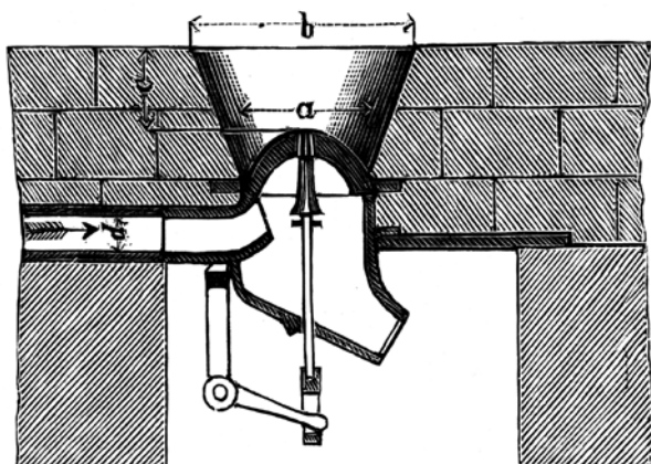
Indmuring af Patent Underblæseren.
