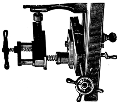
Forsætter til at bore Hullerne i Fælgene — kan stilles i forskjellig Højde.
