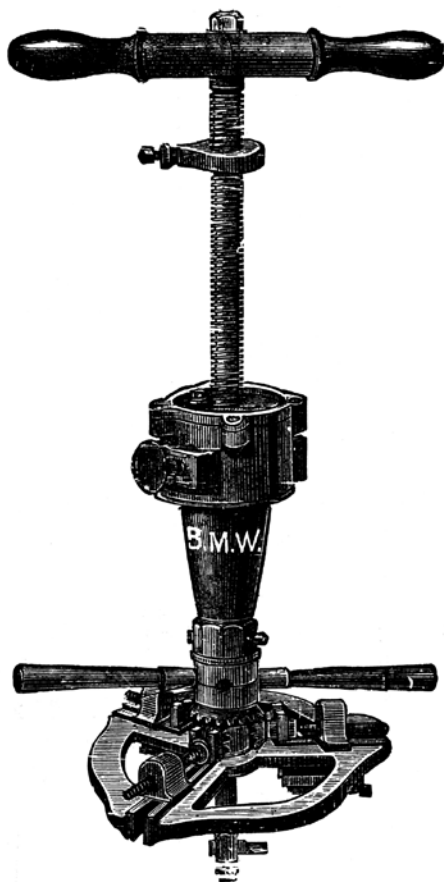
No. 212. til conisk Boring.
