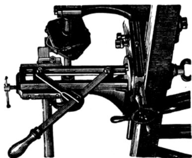
Højdeforsætter til at fraise flade Tapper paa Egerne.
